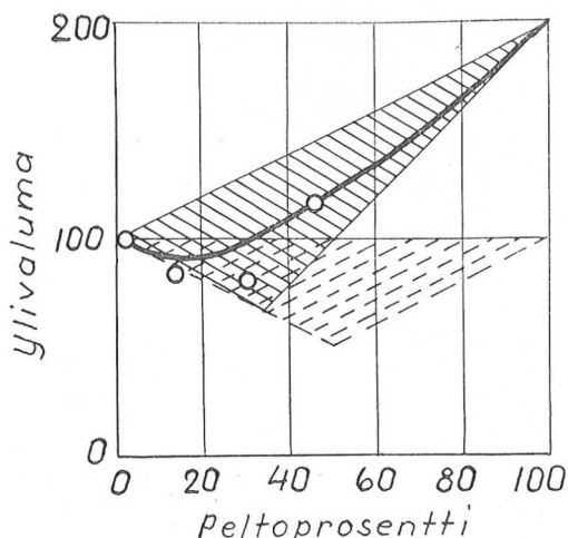
Kuva 2. Ylivaluman riippuvuus peltoprosentista, kun edellytetään, että pellon ylivaluma on kaksinkertainen (ehä viivoitus) tai yhtä suuri (katkoviivoitus) verrattuna metsän ylivalumaan.
